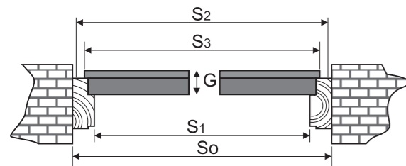
Ajtó függőleges metszet
