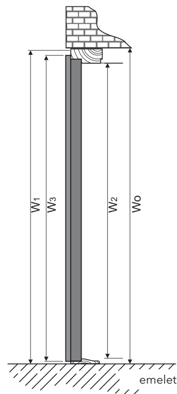
Ajtó vízintes metszet
